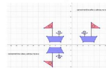
Osnosimetrične slike u odnosu na osi koordinatnog sustava
